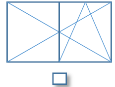
Oscillo-battant 2 vantaux OB2
