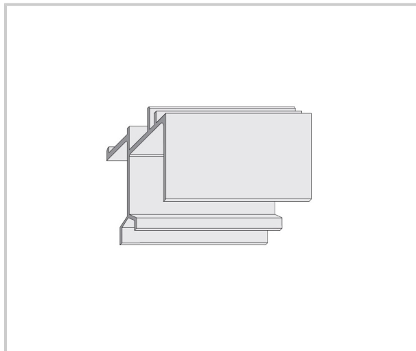
Profil de guidage haut Modèle HH0130
