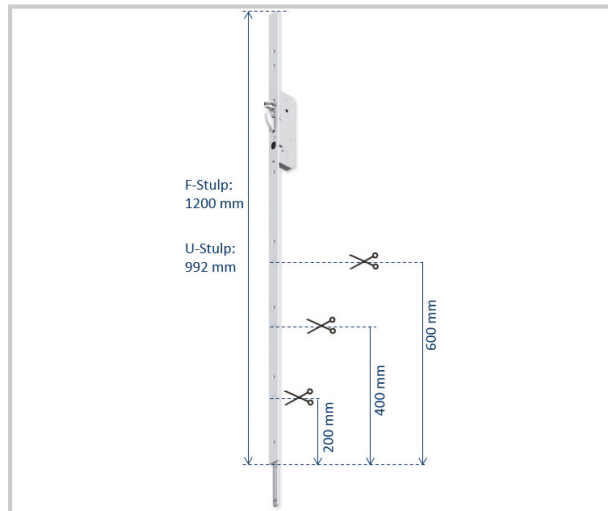
Rallonge serrure U24x6.
